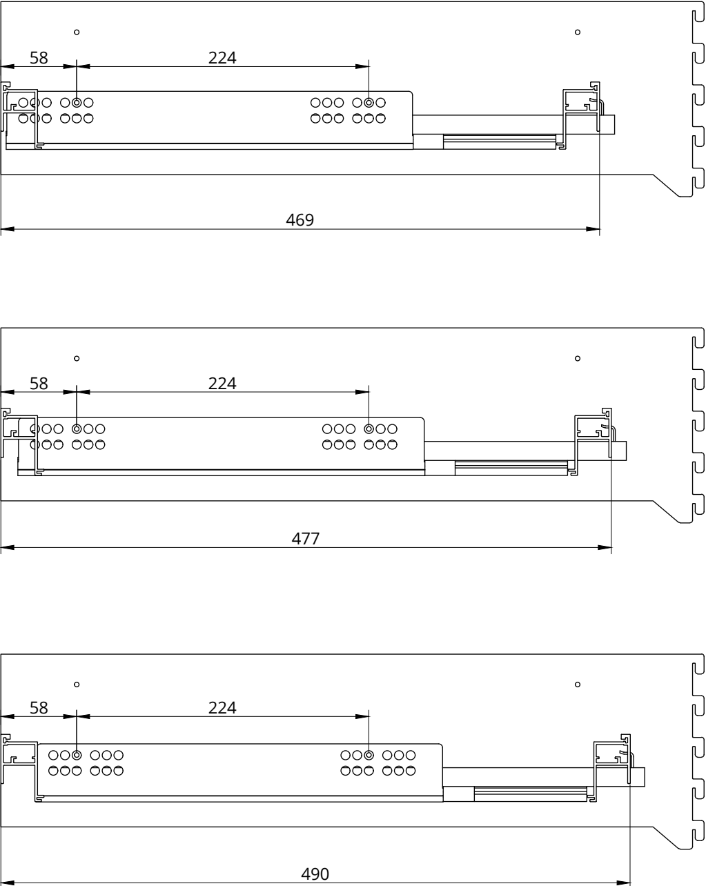
НАПРАВЛЯЮЩАЯ HETTICH QUADRO L 470 MM
