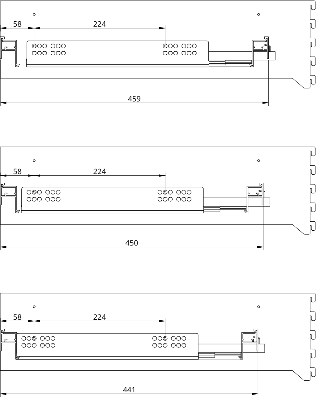
НАПРАВЛЯЮЩАЯ HETTICH QUADRO L 420 MM
