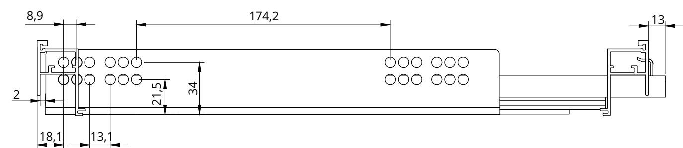
MIXBOX 45, НАПРАВЛЯЮЩАЯ HETTICH QUADRO L 470 MM
