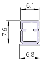
СВЕТОРАССЕИВАЮЩИЙ ПРОФИЛЬ
