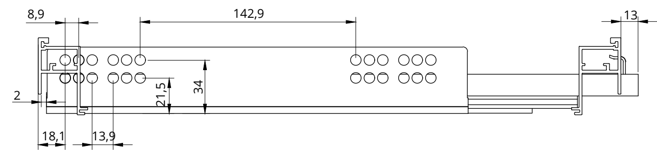
MIXBOX 45, НАПРАВЛЯЮЩАЯ HETTICH QUADRO L 420 MM
