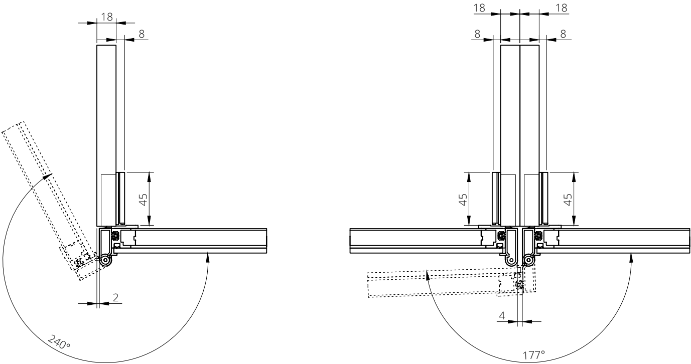
УГОЛ ОТКРЫВАНИЯ ПЕТЛИ FLEX:
