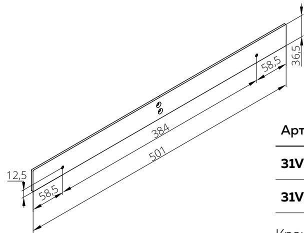
КРОНШТЕЙН НАКЛОННЫЙ 15° ДЛЯ ПОЛКИ
