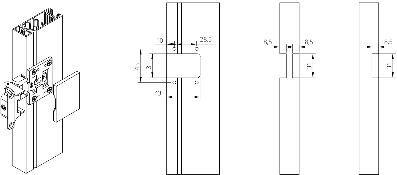
ФРЕЗЕРОВКА ПРОФИЛЯ TETRIX ДЛЯ ПЕТЛИ FLEX:
