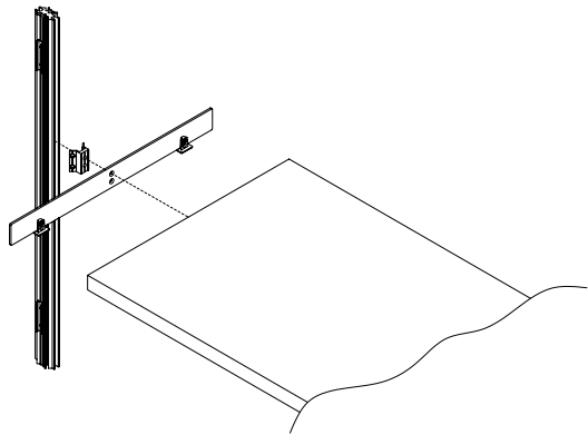
КРЕПЕЖ УНИВЕРСАЛЬНОГО КРОНШТЕЙНА ДЛЯ ПОЛКИ, Н=35 ММ
