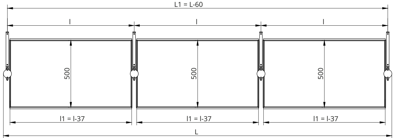
РАСЧЕТ ШИРИНЫ ПОЛКИ
