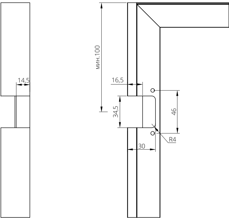
ФРЕЗЕРОВКА ФАСАДА ИЗ ПРОФИЛЯ PIXEL ДЛЯ ПЕТЛИ FLEX:
