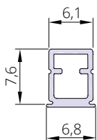
СВЕТОРАСSEИВАЮЩИЙ ПРОФИЛЬ
